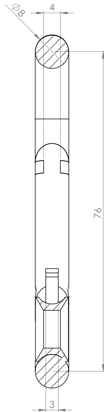
SECTION A-A SCALE 2 : 1
